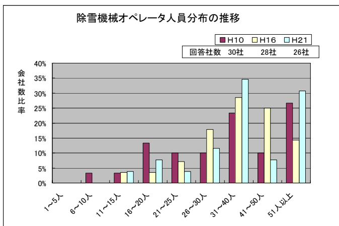
図-10 除雪機械の人員分布の推移(直轄)
