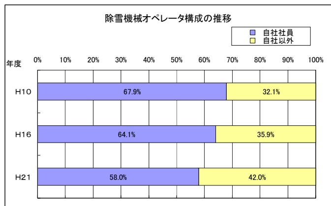
図-11 除雪機械オペレータ構成の推移(直轄)
